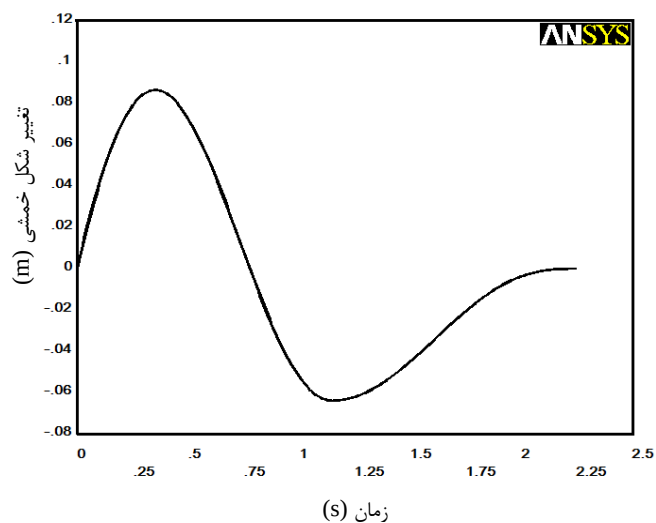
شکل ۱۷- محاسبه تغییر شکل خمشی مقطع (X=۶۶متر) با نرم افزار ANSYS
