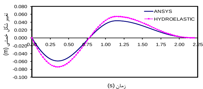
شکل ۱۹ - مقایسه نتایج حاصل از نرم افزار ANSYS و برنامه HYDROELASTIC در محاسبه تغییر شکل خمشی پاشنه کشتی ( X=0 ) در پدیده کوبش سینه
