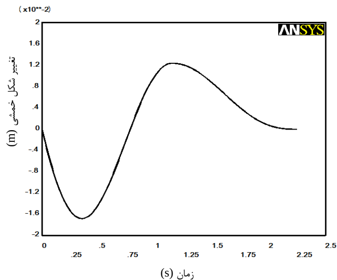
شکل ۱۵- محاسبه تغییر شکل خمشی مقطع (X=۲۲متر) با نرم افزار ANSYS
