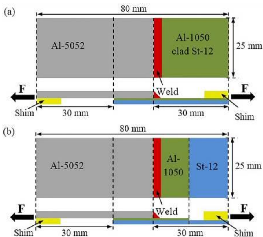
شکل ۳- ابعاد نمونه‌های آزمون کشش-برش که در (a) فولاد St-۱۲ و لایه واسط Al-۱۰۵۰ و در (b) فقط فولاد St-۱۲ در فک دستگاه کشش قرار می‌گیرد
