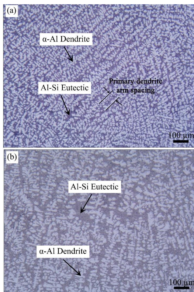
شکل ۸- تصاویر نوری از ریزساختار فلز جوش مربوط به جوش ایجاد شده با حرارت ورودی: (a) 290\ J\ mm^{-1} ، (b) 400\ J\ mm^{-1} .
