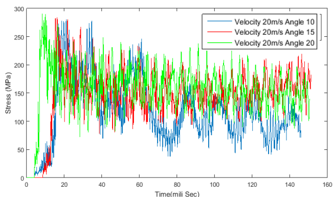
شکل ۱۱- تغییرات تنش پوسته در سرعت اولیه ۲۰ متر بر ثانیه در زاویه‌های برخورد ۱۰، ۱۵ و ۲۰ درجه
