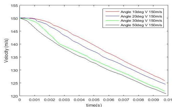
شکل ۴- تغییرات سرعت برخورد با آب بر حسب زمان با تغییر در زاویه برخورد در نرم‌افزار LS-DYNA
