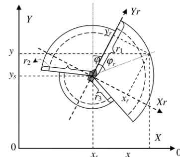
شکل ۶- دامنه ایمن دایره‌ای Goodwin
