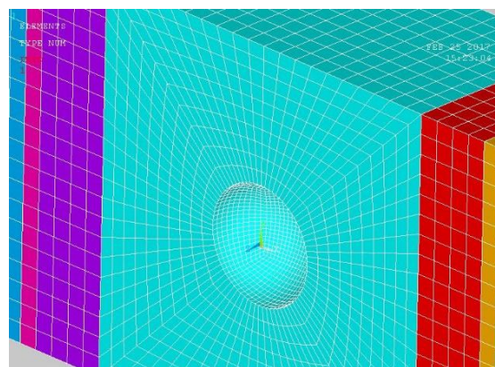
شکل ۱۱- مقطع پوشش جاذب دارای حفره کروی شکل
