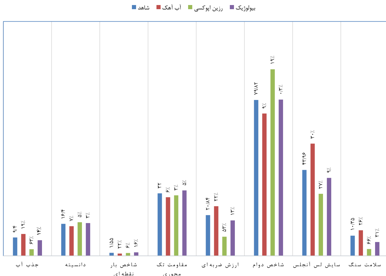
شکل ۸- مقایسه خواص مهندسی نمونه‌های پهنساز شده با نمونه شاهد
