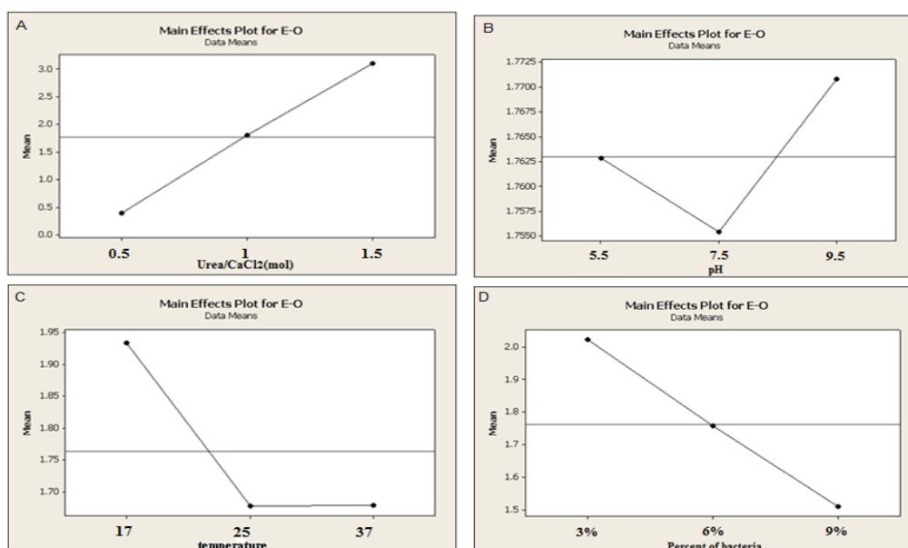
شکل ۵- بررسی تاثیر غلظت اوره و کلرید کلسیم (A)، تاثیر pH (B)، تاثیر دما (C) و تاثیر باکتری (D) در آزمایش‌ها
