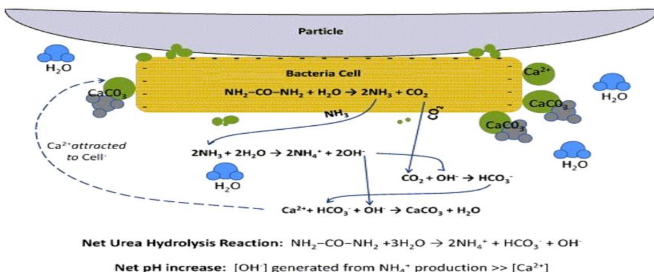
شکل ۷- تصویر شماتیکی از واکنش‌های بیوشیمیایی در ماتریکس خاک [۲۷]
