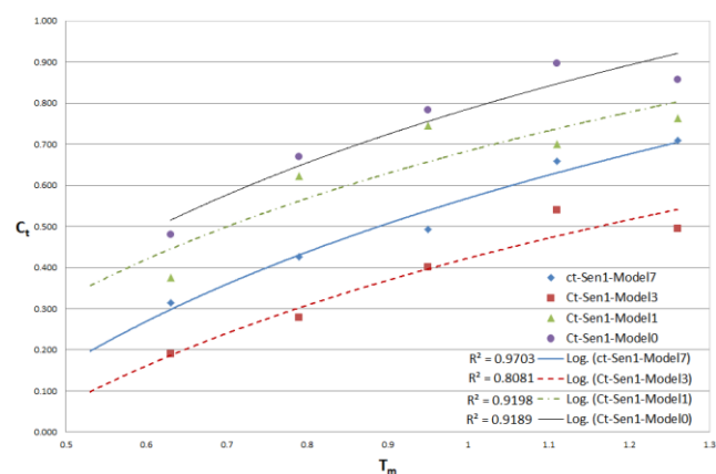
شکل ۸: مقایسه عملکرد مدل های پله ای و دوزنقه ای با مدل مبنا
