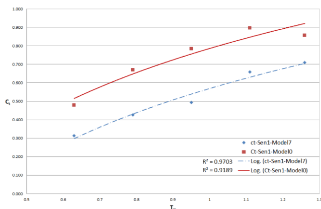
شکل ۷: مقایسه عملکرد موج شکن پله‌ای و مدل مبنا
