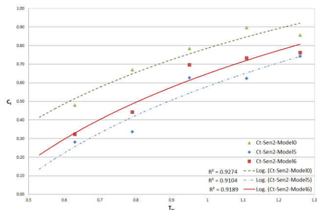
شکل ۱۱: مقایسه موج شکن‌های با مقطع دارای انحنا با نمونه مبنا در شبیه سازی گروه دوم
