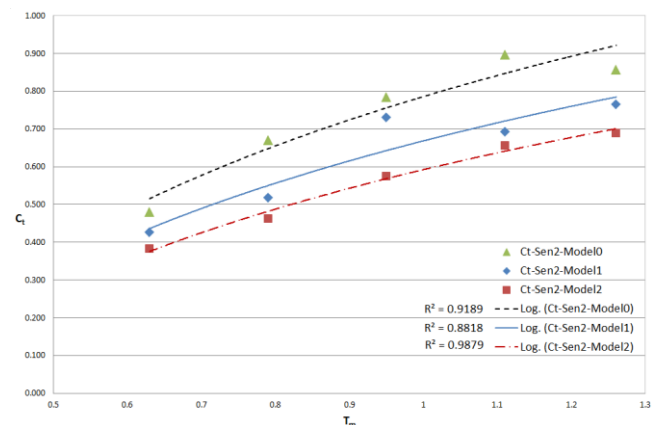
شکل ۹: مقایسه عملکرد نمونه مبنا با نمونه‌های ۱ و ۲ در حالت سطح و جرم برابر
