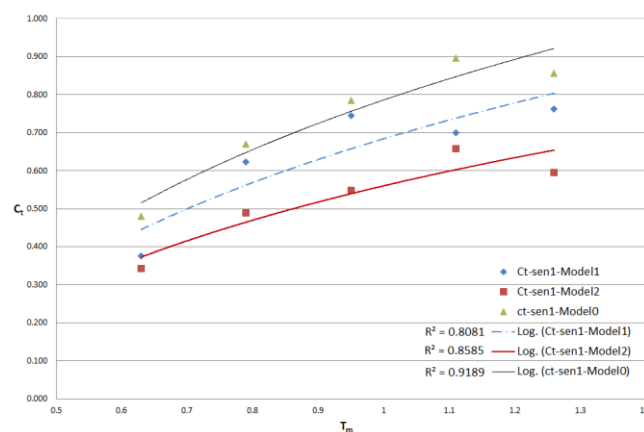
شکل ۴: مقایسه ضریب انتقال در مدل های شماره ۱ و ۲ با مدل مبنا
