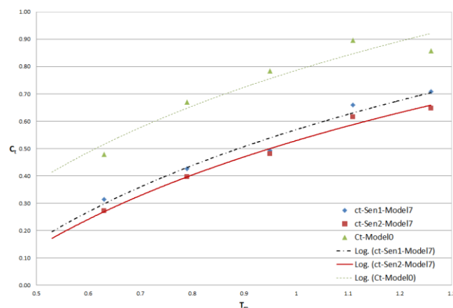
شکل ۱۴: مقایسه عملکرد موج شکن پله ای و مبنا در هر دو شبیه سازی
