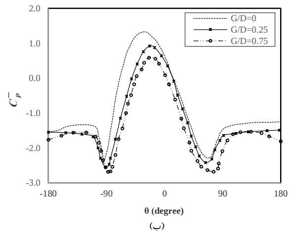
شکل ۴- توزیع مقدار متوسط ضریب فشار بر روی (الف) استوانه اصلی ( Re=0.75 \times 10^4 ) و (ب) استوانه فرعی ( Re=2 \times 10^4 )
