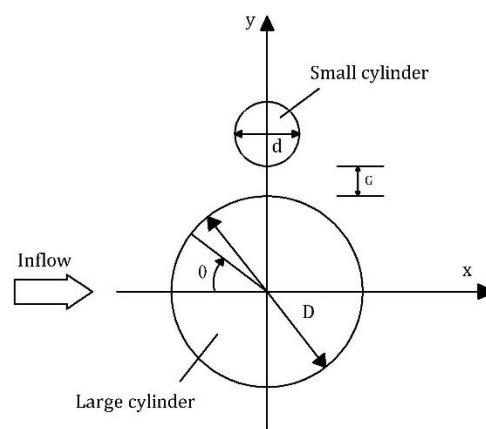
شکل ۱- جزئیات مدل‌های مورد بررسی
