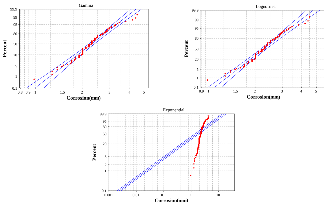
شکل ۵- دیاگرام احتمالاتی در سال ۳۵ عمر سکو در بازه اطمینان ۹۵٪
