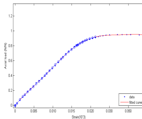
شکل ۴- خروجی نرم افزار برای نمونه [۱۸]
