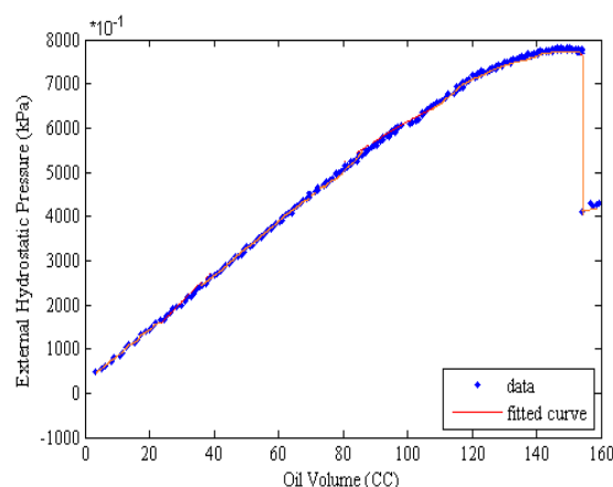
شکل ۱۶- نمودار کماتشی خروجی از نرم افزار برای ضریب (۰/۴)
