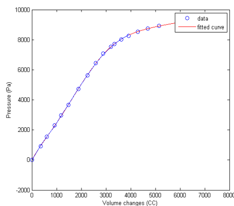
شکل ۵- خروجی نرم افزار برای نمونه [۱۹]
