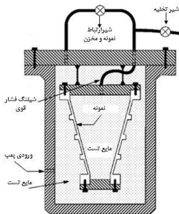
شکل ۷- شماتیک دستگاه آزمایش در روش کنترل حجم [۷]
