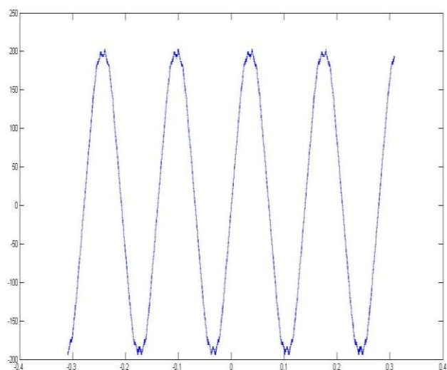
شکل ۱۴ - ولتاژ فاز القایی اندازه‌گیری شده
