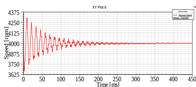
شکل ۹ - شکل موج سرعت موتور BLDC در حالت تحت بار
