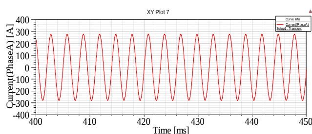
شکل ۱۰ - شکل موج جریان موتور BLDC در حالت بارداری
