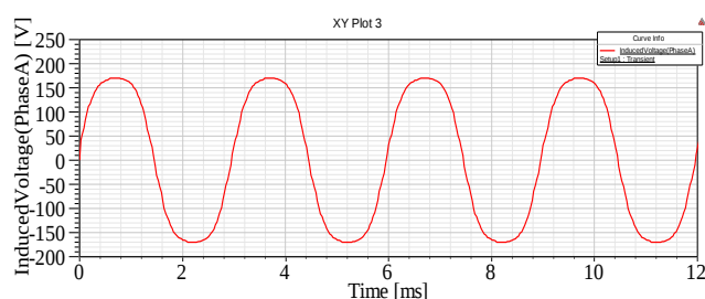
شکل ۷ - شکل موج Back-EMF هر فاز
