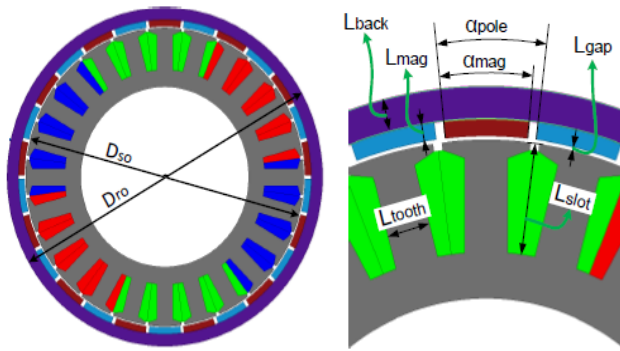
شکل ۴ - ساختار دندانه و شیار و توپولوژی دو بعدی موتور مغناطیس دائم رتور خارجی [۲۸]
