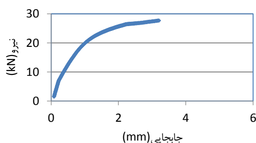
شکل ۲۶- نمودار تست کشش نمونه W۳.
