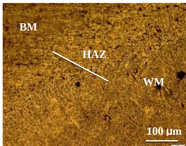
شکل ۱۱- تصویر ریز ساختار فصل مشترک نمونه W۱.
