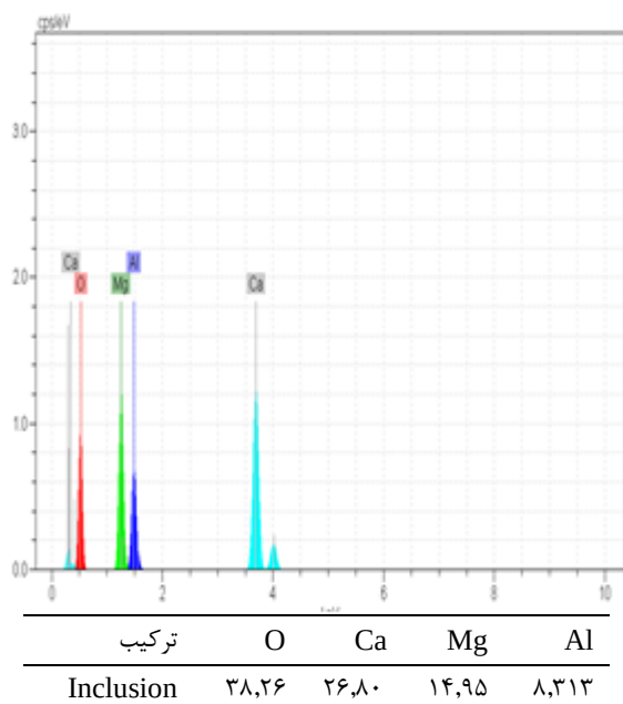
شکل ۲۰- نتایج آنالیز رسوب B، در منطقه متاثر از حرارت نمونه W۳.
