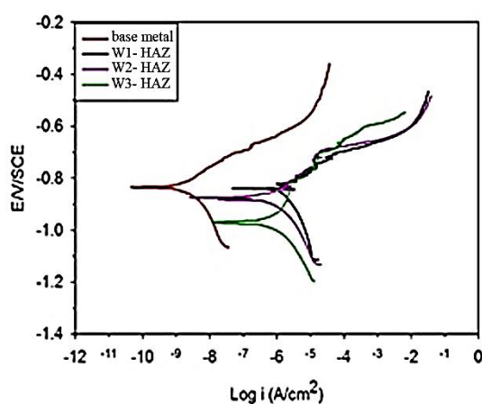
شکل ۳۳- نمودار خوردگی پلاریزاسیون پتانسیودینامیک منطقه متأثر از حرارت نمونه‌ها.
