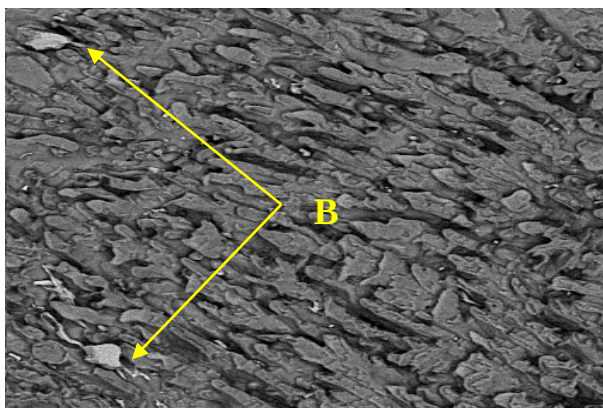
شکل ۱۶- تصویر میکروسکوپ الکترونی از منطقه متأثر از حرارت نمونه W۲.
