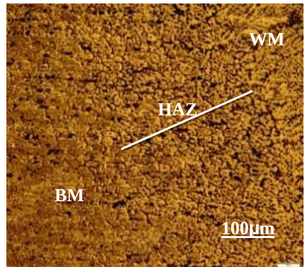
شکل ۱۲- تصویر ریز ساختار فصل مشترک نمونه W۲.
