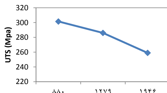
شکل ۲۷- نمودار میانگین استحکام نهایی نسبت به حرارت ورودی.
