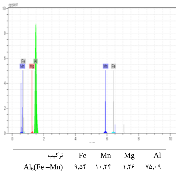
شکل ۱۵- نتایج آنالیز رسوب در منطقه متأثر از حرارت نمونه W۱.
