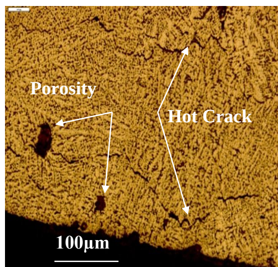
شکل ۲۲- تصویر ریز ساختار عیوب جوش نمونه W۳.
