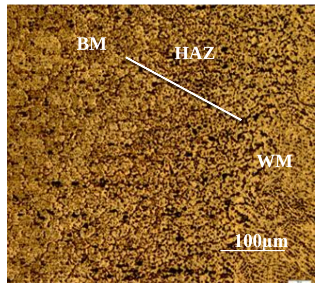
شکل ۱۳- تصویر ریز ساختار فصل مشترک نمونه W۳.
