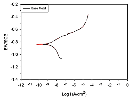
شکل ۳۱- نمودار خوردگی پلاریزاسیون پتانسیودینامیک برای فلز پایه.
