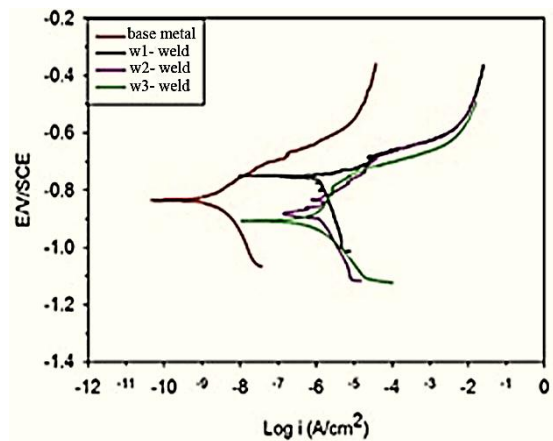
شکل ۳۲- نمودار خوردگی پلاریزاسیون پتانسیودینامیک منطقه جوش برای همه‌ی نمونه‌ها در کنار فلز پایه.
