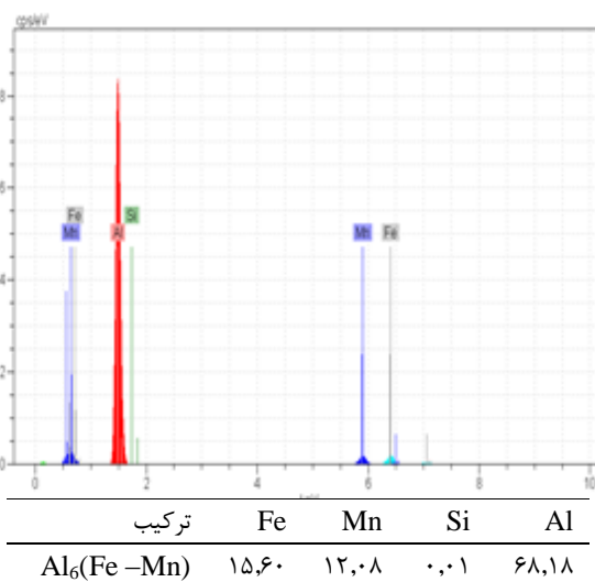
شکل ۱۷- نتایج آنالیز رسوب در منطقه متاثر از حرارت نمونه W۲.
