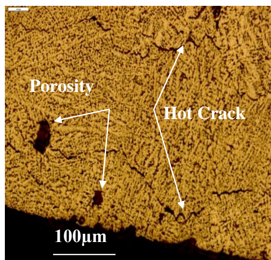
شکل ۲۲- تصویر ریز ساختار عیوب جوش نمونه W3.
