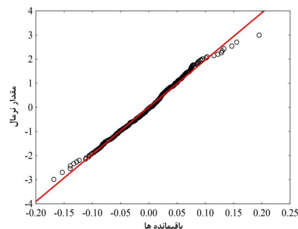
شکل ۱۶- نمودار احتمال نرمال برای باقیمانده‌های مدل نهایی انزلی
