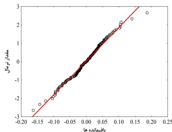
شکل ۱۵- نمودار احتمال نرمال برای باقیمانده‌های مدل نهایی نوشهر
