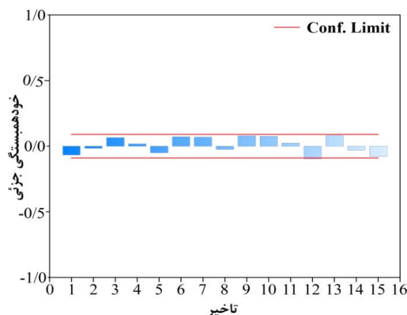
شکل ۱۴- خودهمبستگی جزئی برای باقیمانده‌های مدل نهایی انزلی
