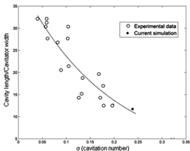
شکل ۳- تغییرات طول بی بعد کاواک بر اساس عدد کاواکری برای کاواک‌های نوع سهموی [۲۰]
