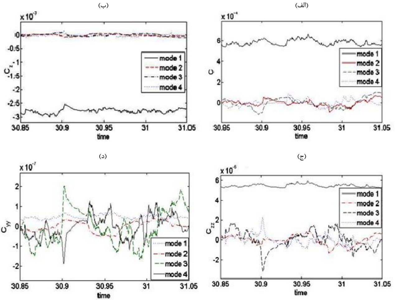
شکل ۷- شدت منابع در مدهای مختلف، (الف): تک قطبی، (ب): دو قطبی، (ج): چهار قطبی خطی در راستای z ، (د): چهار قطبی خطی در راستای y
