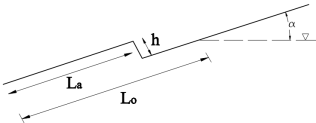
شکل ۱- هندسه مدل ورق پروازی پله‌دار
