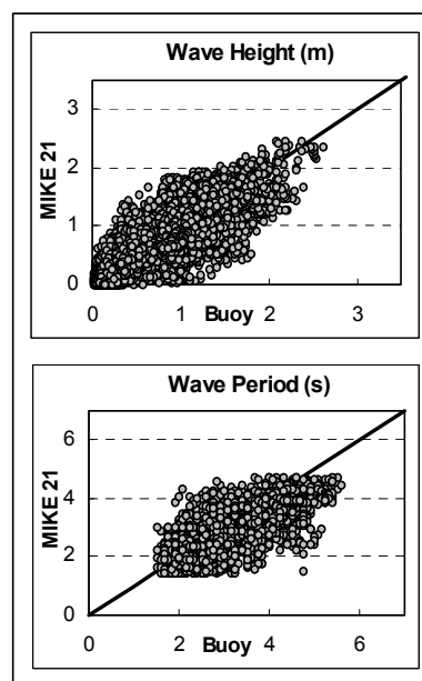
شکل ۱۱- مقایسه مقادیر اندازه‌گیری شده و پیش‌بینی شده ارتفاع و دوره تناوب موج توسط روش عددی (منطقه بوشهر)
