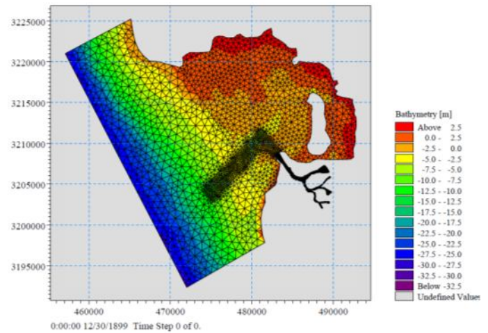
شکل ۱۵- شبکه‌بندی انتخاب شده جهت مدل‌سازی محلی جریان‌های جزر و مدی
