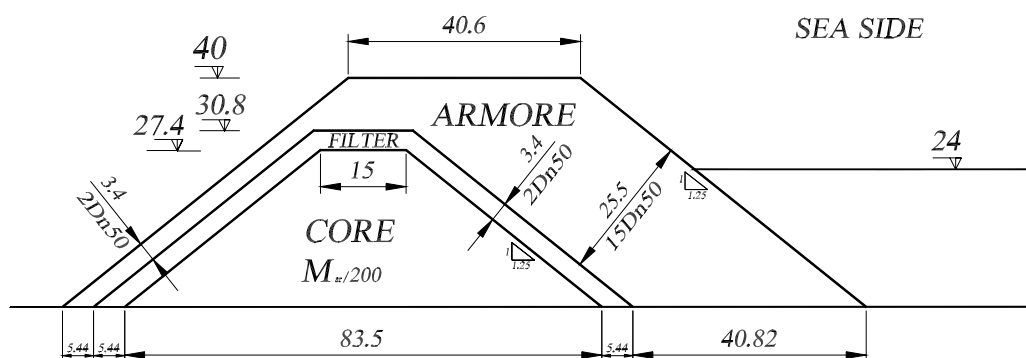
شکل ۱- نمونه مقطع عرضی مدل آزمایشگاهی موج شکن شکل پذیر مورد آزمایش
