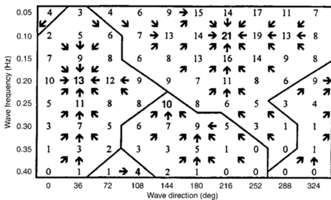
شکل ۱- توزیع انرژی در طیف موج جهت‌دار، افزایندهای آن و نیز محل ماکزیم‌های نسبی [۱۷]
