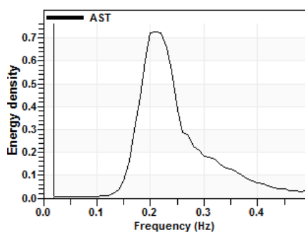
شکل ۳- طیف تک جهته طوفان منتخب ایستگاه شماره ۳ (ارتفاع موج مشخصه ۱/۱۵ متر، پر یود پیک ۴/۷۷ و تاریخ رخداد ۲۰۰۹/۱۱/۲۲)
