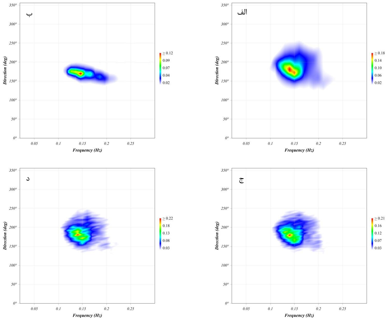
شکل ۱۱- عملکرد توزیع های جهت استاندارد دونلن و همکاران، کالیبره شده و کاملاً کالیبره شده هایپربولیکی در مقایسه با میدانی (رخداد از سمت غرب (\theta_0 = 180^\circ) مورخه ۲۰۱۰/۱۲/۱۳) الف: توزیع جهت میدانی، ب: توزیع جهت دونلن و همکاران [۶] ج: توزیع جهت هایپربولیکی کالیبره شده د: توزیع جهت هایپربولیکی کاملاً کالیبره شده
