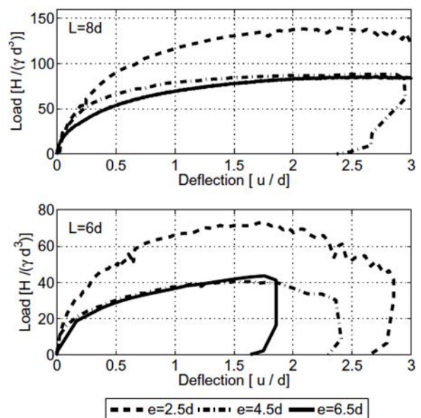
شکل ۷- نمودارهای نیرو- تغییر مکان سرشمع در طول آزاد و عمق مدفون‌های متفاوت [۱۴]
