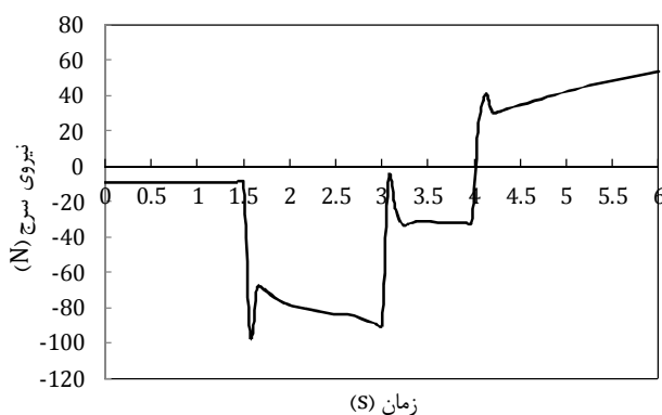
شکل ۱۶- نمودار تغییرات نیروی سرچ در حرکت شتابدار سرچ
