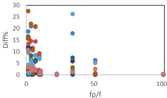
شکل ۱۲: درصد اختلاف عکس العمل تکیه‌گاهی در دو روش با اندرکنش و بدون اندرکنش در سه جهت برحسب نسبت فرکانسی سیستم ثانویه به سازه اصلی
