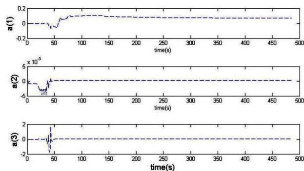
شکل ۷: ضرائب a_1 و a_2 و a_3 محاسبه شده از روش شناسایی سیستم
