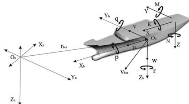
شکل ۱- مختصات ثابت و متحرک در حرکت شناور [۱۷]
