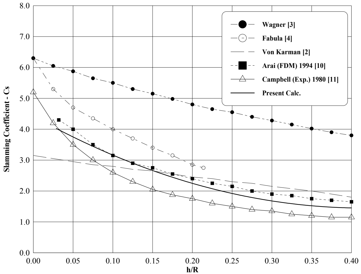
شکل ۲- تغییرات ضریب نیروی برخورد با آب بر حسب h/R ( سرعت برخورد 10 \text{ m/s} و شعاع استوانه 5/5 \text{ m} )
