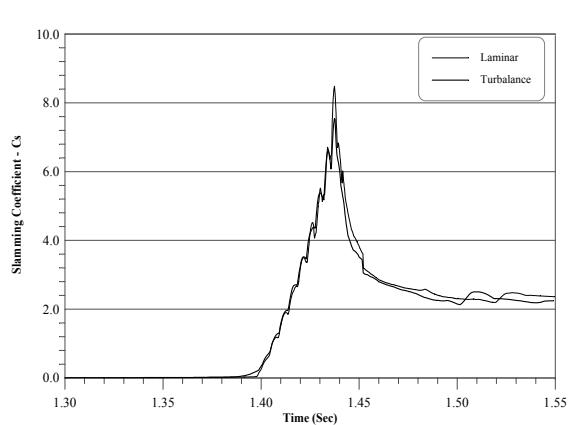
شکل ۹- تغییرات ضریب نیروی برخورد با آب بر حسب زمان
