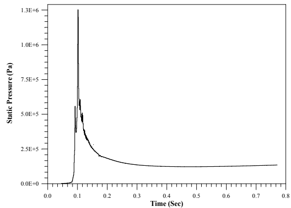
شکل ۳- نمودار فشار در پایین ترین نقطه استوانه بر حسب زمان
