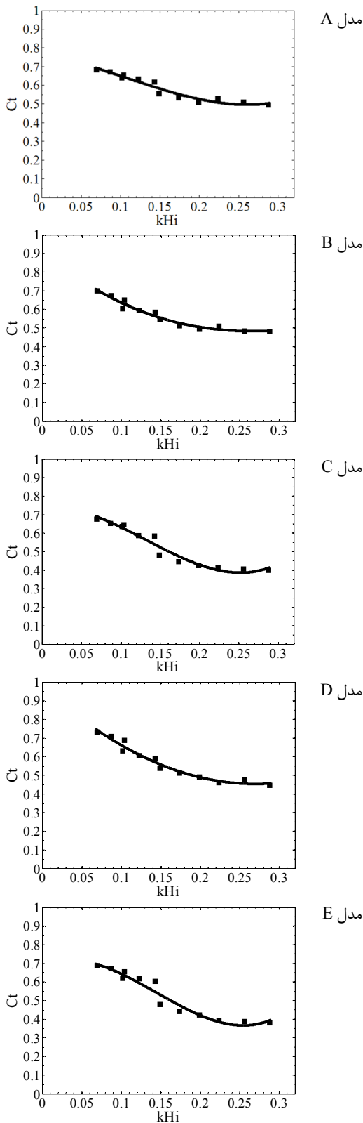
شکل ۸- عملکرد هیدرودینامیکی مدل‌های
