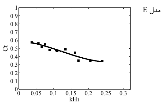
شکل ۹- عملکرد هیدرودینامیکی مدل‌های
