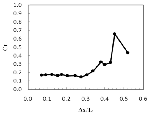
شکل ۲- تغییرات ضریب انعکاس با فاصله بین موج‌نگارها
