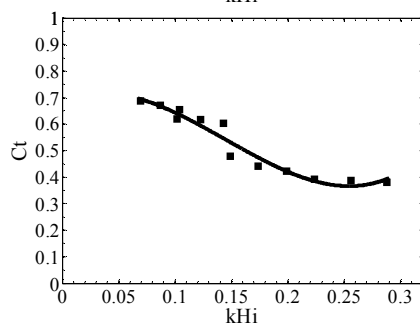
شکل ۸- عملکرد هیدرودینامیکی مدل‌های
