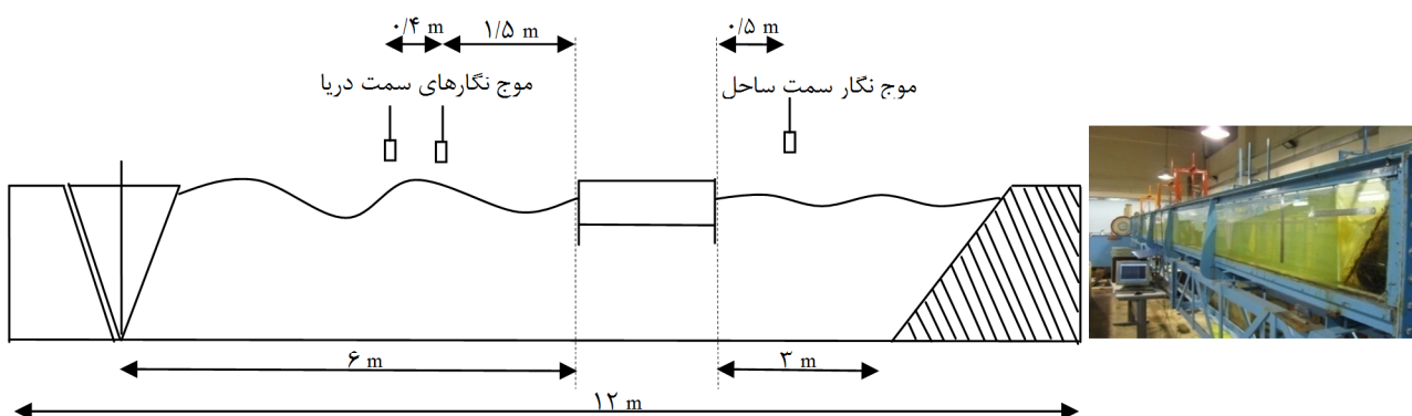
شکل ۱- نمای کلی فلوم موج‌ساز، مخزن موج (راست)، جانمایی تجهیزات آزمایشگاهی (چپ)
