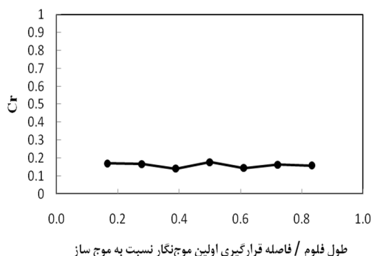
شکل ۳- تغییرات ضریب انعکاس نسبت به موقعیت موج‌نگارها در فلوم
