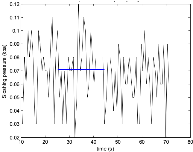
شکل ۱۴- فشار اسلاشینگ با ارتفاع آب درون مخزن ۲ سانتیمتر که توسط حسگر شماره ۵ در امواج از پهلو ثبت شده؛ فرکانس و دامنه حرکت هیو و پیچ شناور به ترتیب ۱ سیکل بر ثانیه، ۲ سانتیمتر و ۲/۵ درجه
