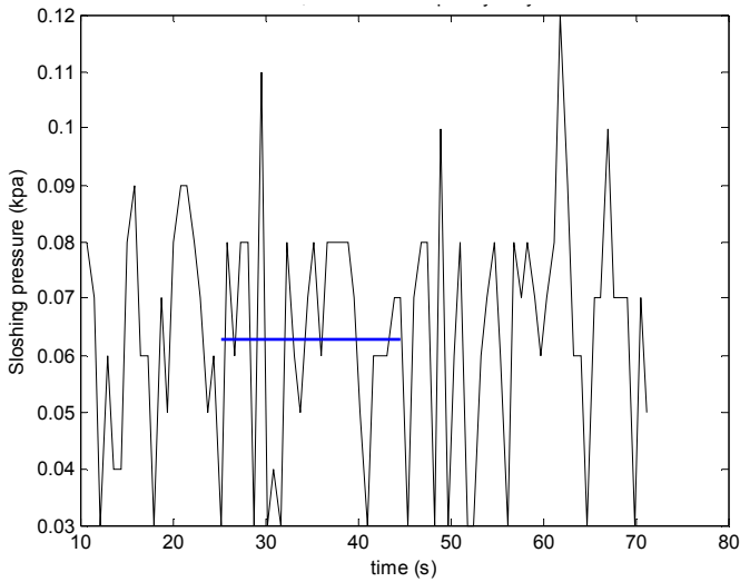
شکل ۱۳- فشار اسلاشینگ با ارتفاع آب درون مخزن ۲ سانتیمتر که توسط حسگر شماره ۱ در امواج از پهلو ثبت شده؛ فرکانس و دامنه حرکت هیو و پیچ شناور به ترتیب ۱ سیکل بر ثانیه، ۲ سانتیمتر و ۲/۵ درجه
