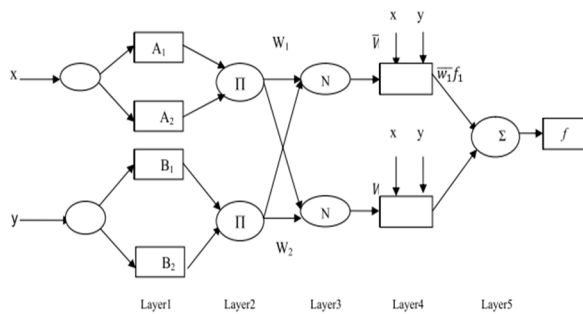
شکل ۳- ساختار سامانه استنتاج تطبیقی عصبی- فازی (ANFIS)
