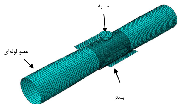
شکل ۵- نمایی کلی از هندسه مدل و نحوه‌شن‌بندی
