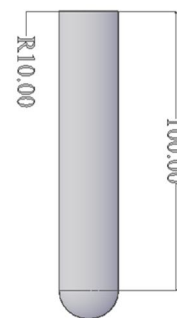
شکل ۳- مشخصات هندسی سنبه (واحد mm)
