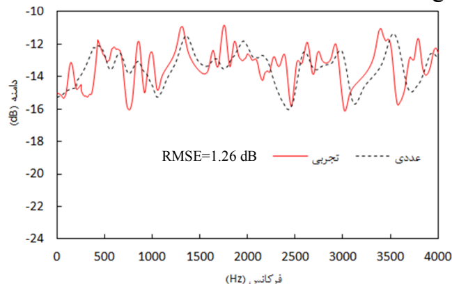
شکل ۳- مقایسه دامنه توابع پاسخ فرکانسی سیستم اولیه برای سه نقطه (الف) SL1، (ب) SL4 و (ج) SP2
