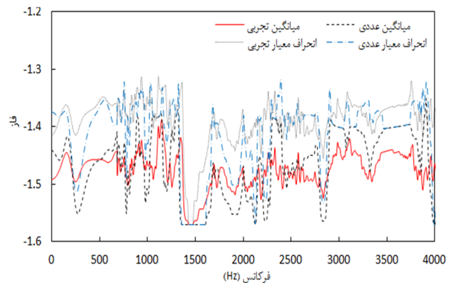
شکل ۹. مقایسه میانگین و انحراف معیار فاز تابع پاسخ فرکانسی نقطه SL4
