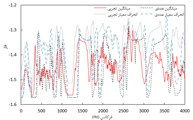
شکل ۱۰. مقایسه میانگین و انحراف معیار فاز تابع پاسخ فرکانسی نقطه SP2
