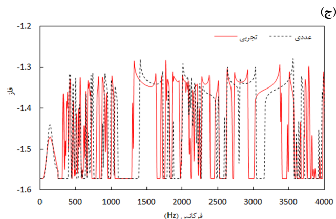
شکل ۷- مقایسه فاز توابع پاسخ فرکانسی سیستم اولیه برای سه نقطه (الف) SL1، (ب) SL4 و (ج) SP2
