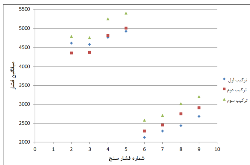
شکل ۸- مقدار فشار میانگین محاسبه شده با استفاده از نتایج مدل عددی برای تمام فشارسنجها در ترکیب متفاوت ارتفاع و پریود موج
