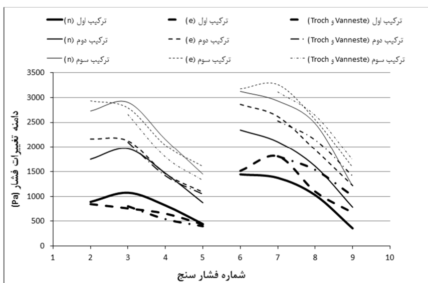
شکل ۷- دامنه تغییرات فشار برحسب پاسکال در هر محل هر یک از فشارسنجها برای سه ترکیب متفاوت ارتفاع و پریود موج (خط ممتد = نتایج مدل عددی، خط چین = نتایج مدل آزمایشگاهی، خط و نقطه = رابطه Troch و Vanneste)
