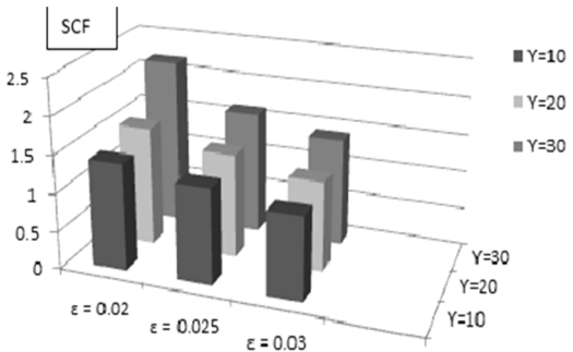
شکل ۱۵- تأثیر ناکاملی هندسی عضو مهارى روی SCF در (α = 12, β = 0.6 θ = 90°, τ = 0.4) Crown 0°
