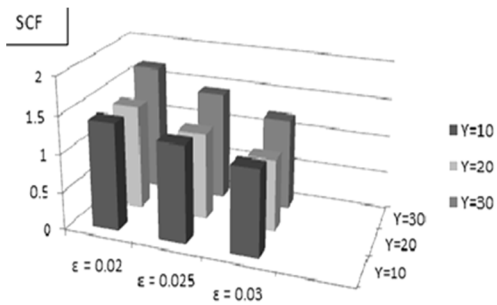
شکل ۱۴- تأثیر ناکاملی هندسی عضو مهارى روی SCF در (α = 12, β = 0.45, θ = 90°, τ = 0.4) Crown 0°
