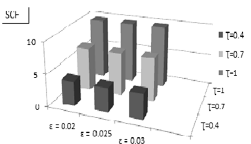
شکل ۱۰- تأثیر ناکاملی هندسی عضو مهارى روی SCF در (α = 12, θ = 90°, β = 0.3, γ = 10) Saddle
