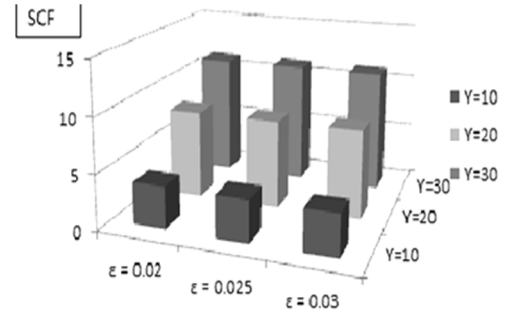
شکل ۸- تأثیر ناکاملی هندسی عضو مهارى روی SCF در (α = 12, β = 0.45, θ = 90°, τ = 0.4) Saddle
