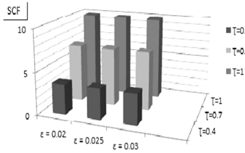
شکل ۱۲- تأثیر ناکاملی هندسی عضو مهارى روی SCF در (α = 12, β = 0.6, θ = 90°, γ = 10) Saddle
