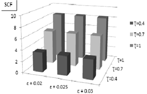
شکل ۱۰- تأثیر ناکاملی هندسی عضو مهارى روی SCF در (α = 12, θ = 90°, β = 0.3, γ = 10) Saddle
