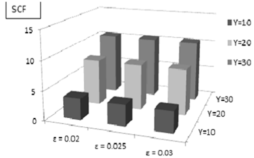
شکل ۹- تأثیر ناکاملی هندسی عضو مهارى روی SCF در (α = 12, β = 0.6, θ = 90°, τ = 0.4) Saddle
