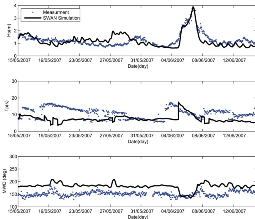
شکل ۴- مقایسه بین ارتفاع موج شاخص، پریود پیک و جهت متوسط موج اندازه گیری شده و شبیه سازی شده در دستگاه AW1
