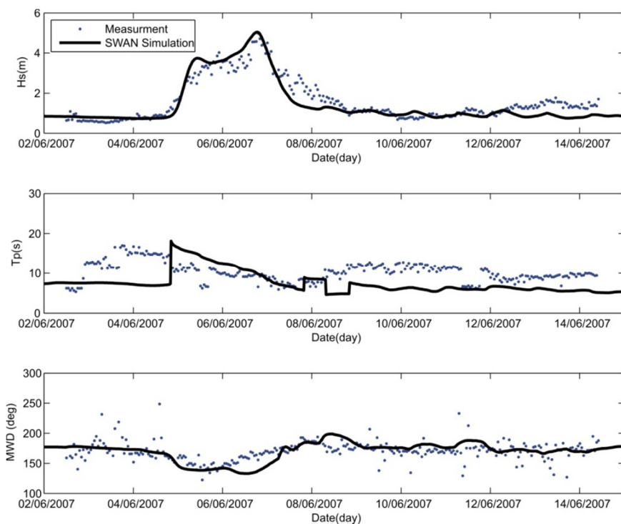
شکل ۵- مقایسه بین ارتفاع موج شاخص، پریود پیک و جهت متوسط موج اندازه گیری شده و شبیه سازی شده در دستگاه AW2
