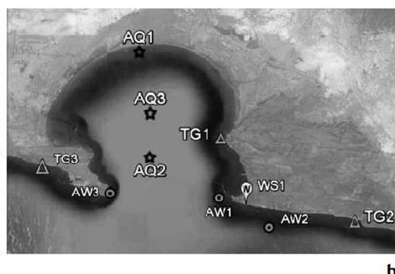
شکل ۲- موقعیت دستگاههای اندازه گیری در خلیج چابهار حین وقوع توفان گنو
