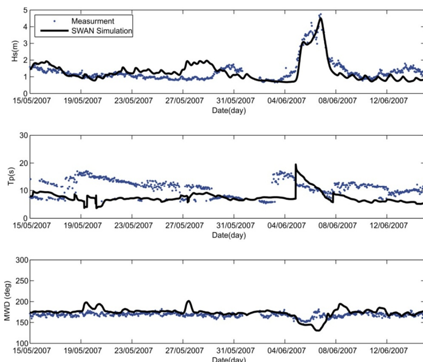
شکل ۶- مقایسه بین ارتفاع موج شاخص، پریود پیک و جهت متوسط موج اندازه گیری شده و شبیه سازی شده در دستگاه AW3
