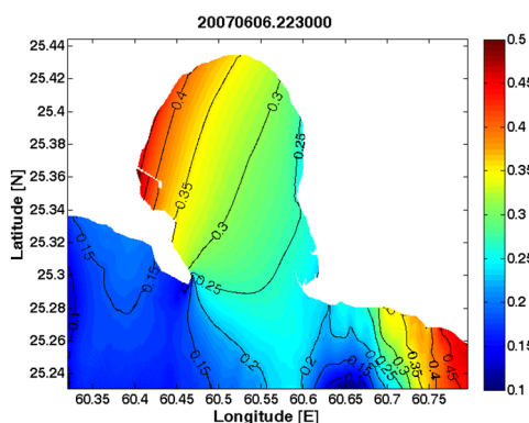
شکل ۱۱- تغییر تراز مد بیشینه ناشی از توفان گنو در خلیج چابهار
