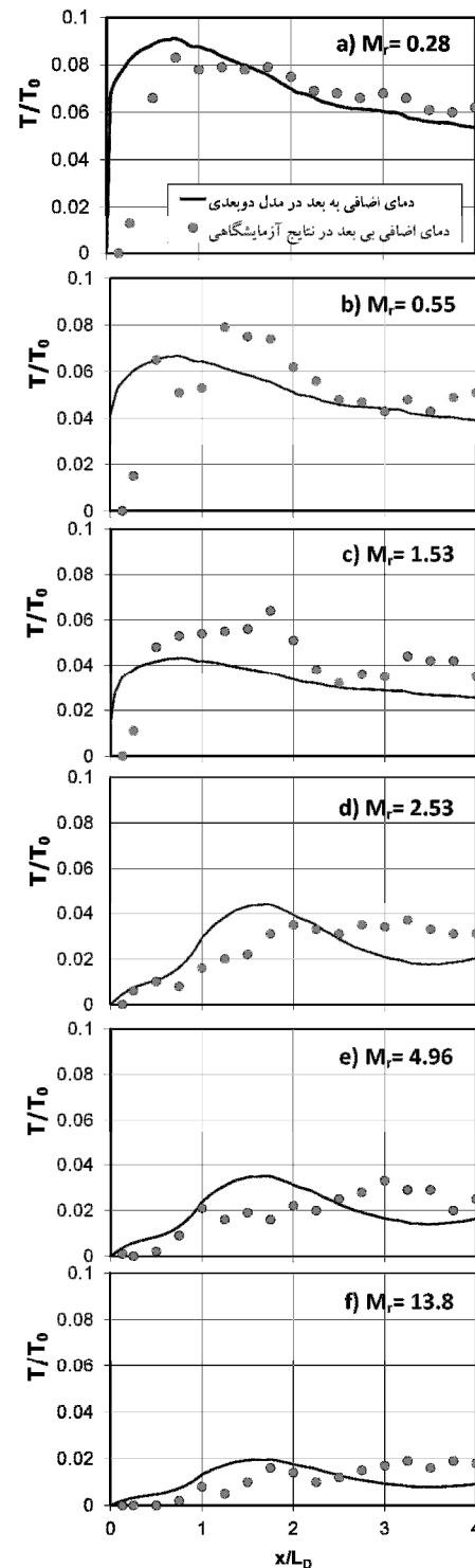
شکل ۶- دمای اضافی ۱۸ بی‌بعد طولی در مرکز پخش‌انده‌ها در کانال آزمایشی، مشاهدات آزمایشگاهی و حل دو بعدی میانگین عمقی نرم افزار NASIR
