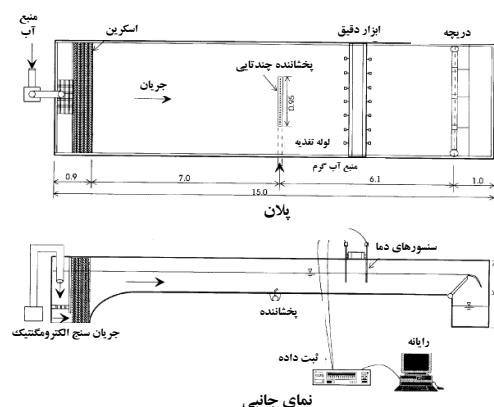
شکل ۵- هندسه و مشخصات کانال آزمایش [۲]
