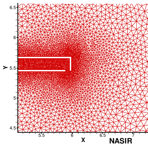
شکل ۷- شبکه‌بندی بی‌ساختار مورد استفاده برای مدل جریان و پخش حرارت (واحدهای مختصات بر حسب کیلومتر می‌باشند و حداقل بعد مثلث ۵ متر تا حداکثر بعد مثلث ۵۰۰ متر)
