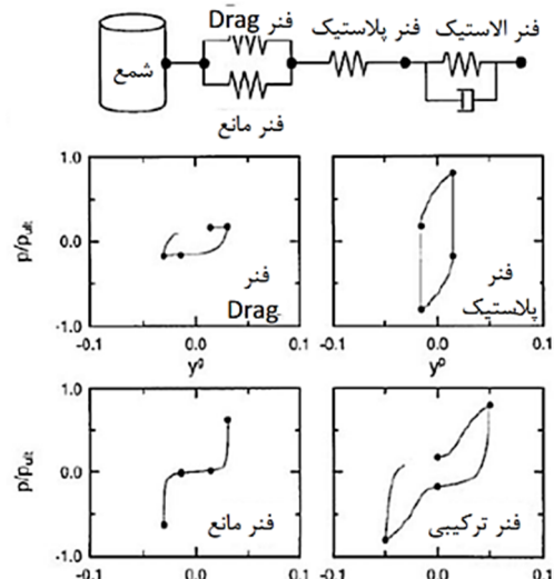
شکل ۷- اجزای تشکیل دهنده ی المان P-y [۱۰]
