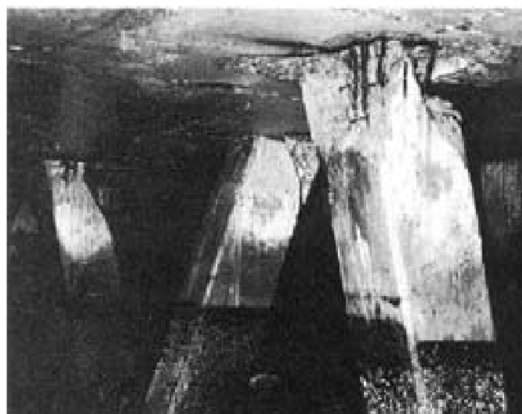
شکل ۱- شمع‌های مایل آسیب دیده در پایانه 7th Street بندر اکلند [۱]
