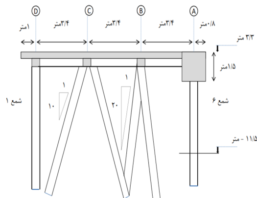
شکل ۲- مقطع عرضی اسکله بازرگانی مورد مطالعه [۸]
