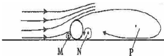
شکل ۱- طرح شماتیک نواحی جدایی در بالادست و پایین دست خط لوله واقع بر بستر [۴]
