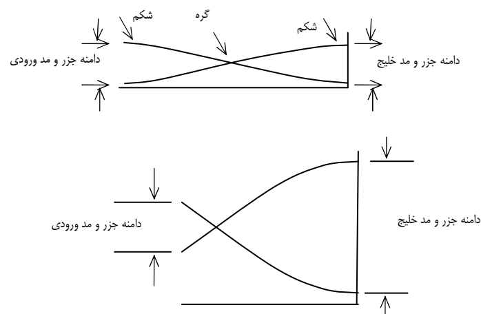
شکل ۳- افزایش دامنه جزر و مد ناشی از پدیده تشدید
