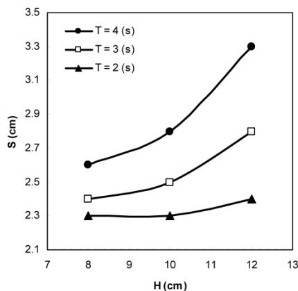
شکل ۳- میزان آبشستگی پنجه موج شکن ( h = 54 (cm), \alpha = 1:0 +/۶۶)
