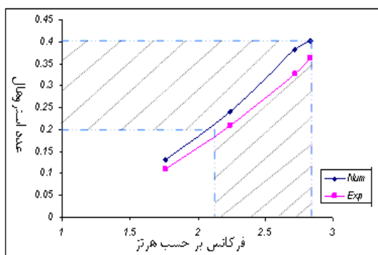
شکل ۲۱- نمودار عدد استروهال بر حسب فرکانس دم زدن
