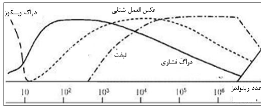
شکل ۱۴- نیروهای وارده بر مدل ماهی
