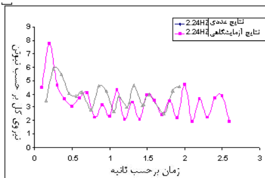
شکل ۲۴- مقایسه نیرو برآیند در جهت X در دو حالت عددی و تجربی (الف) فرکانس ۲.۸۳ هرترتز (ب) فرکانس ۲.۲۴ هرترتز
