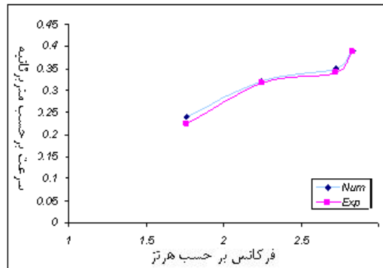
شکل ۲۲- نمودار سرعت بر حسب فرکانس دم زدن
