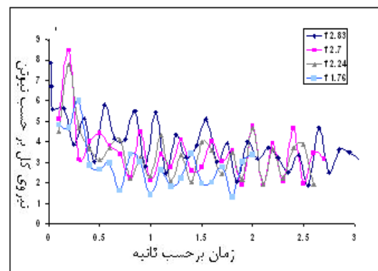
شکل ۲۵- نمودار نیرو برآیند در جهت X بر حسب زمان حاصل از نتایج عددی در دو فرکانس تست شده
