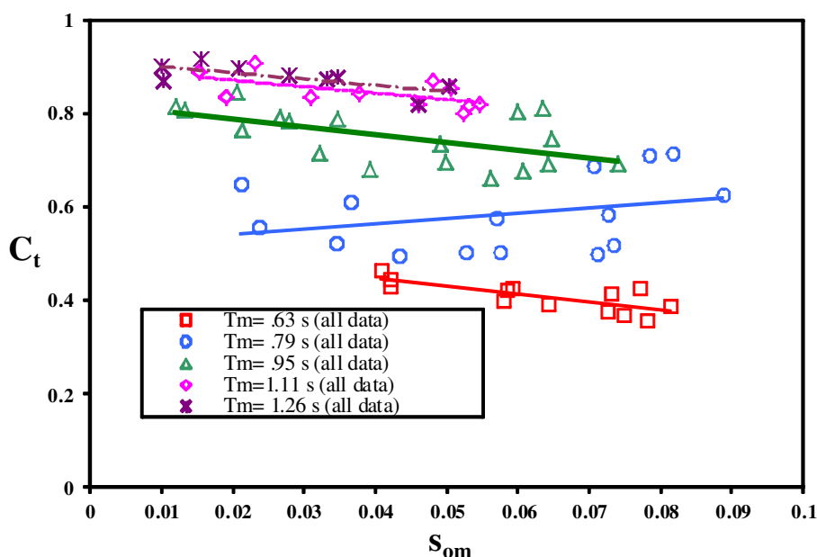
شکل ۳- ضریب انتقال موج برحسب تیزی موج برای موج شکن پانتونی در تمام آبخورها با تفکیک پیوند موج
