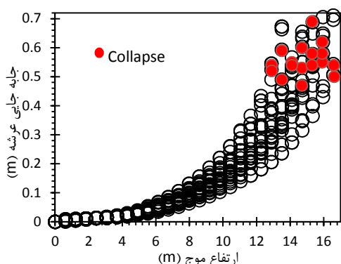
شکل ۸- مقادیر ۲۰ سری تحلیل چندگانه نواری به کمک مدل موج‌نو مقیدشده افزایشی، حاصل از ۲۰×۱۷ تحلیل (بر حسب جابه‌جایی عرشه)
