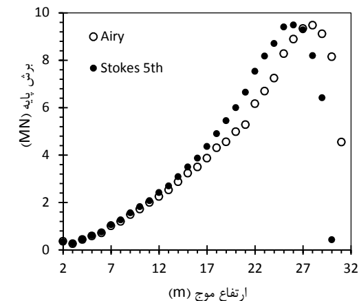
شکل ۱۱- منحنی‌های نواری تحلیل موج افزایشی با استفاده از تئوری امواج منظم ایری و استوکس مرتبه ۵.
