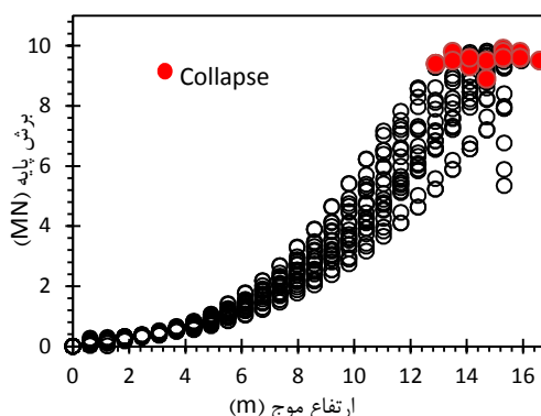
شکل ۹- مقادیر ۲۰ سری تحلیل چندگانه نواری به کمک مدل موج‌نو مقیدشده افزایشی، حاصل از ۲۰×۱۷ تحلیل (بر حسب برش پایه)
