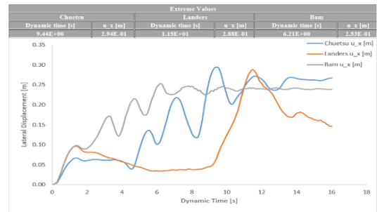
شکل ۴- تغییرات جابه جایی افقی تاج موج شکن کیسونی
