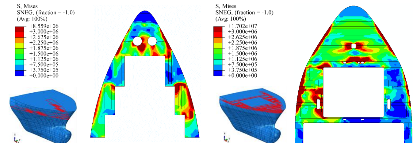
شکل ۲۲- توزیع تنش معادل در مقاطع افقی در ۱/۵ ثانیه - پاسکال.
