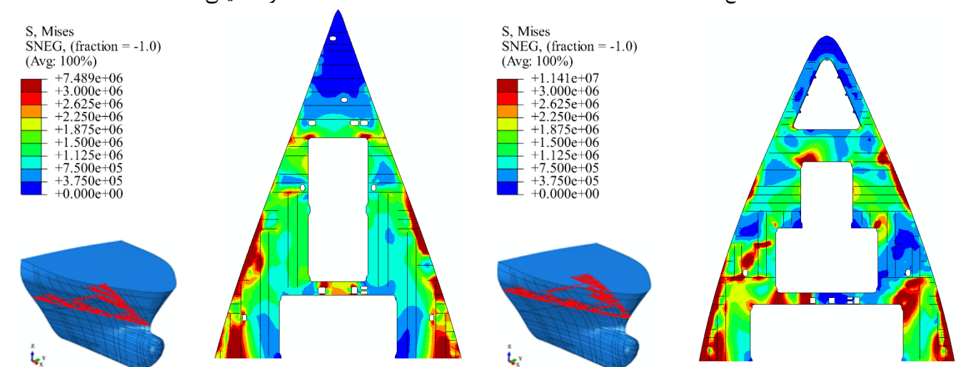
عرشه میانی
