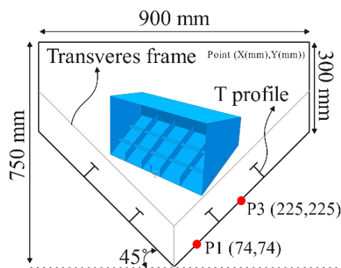
شکل ۹- صفحه عرضی مدل سازی گوه [۲۲].
