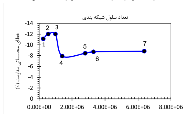
شکل ۹- خطای محاسباتی مقاومت-تعداد سلول های شبکه بندی
