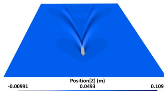
شکل ۱۰- نمایی از سطح آزاد شبیه سازی شده در آب آرام
