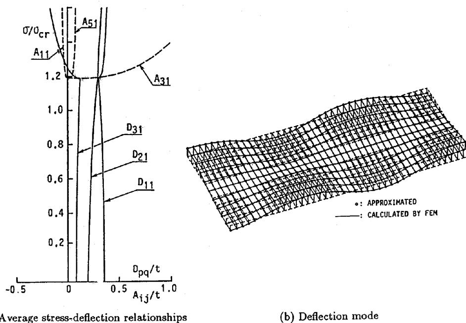
شکل ۳- مؤلفه های تغییرشکلی و مود کمانشی یک ورق ممتد از کف کشتی فله بر، واقع در معرض ترکیب فشار جانبی و تنشهای درون صفحه ای طولی ( h = 30 m )
