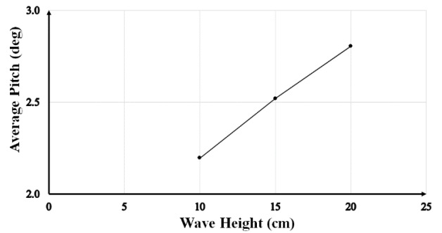
شکل ۱۶- متوسط حرکت پیچ با تغییرات ارتفاع موج در سرعت 5/22 متر بر ثانیه در \lambda/L = 2
