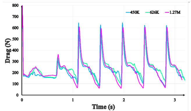
شکل ۷- تاریخچه نیروی پسا با زمان برای ۳ شبکه انتخابی
