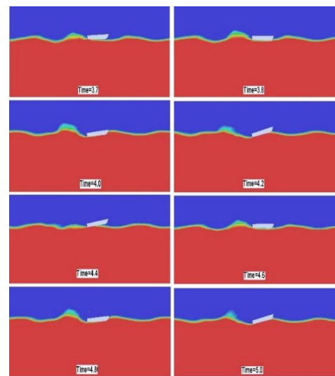
شکل ۸- نمونه‌ای از حرکت شناور در موج در زمانهای
