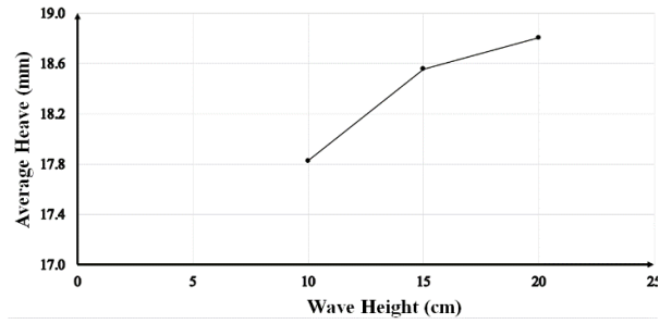
شکل ۱۵- متوسط حرکت هیو با تغییرات ارتفاع موج در سرعت 5/22 متر بر ثانیه در \lambda/L = 2
