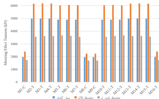
شکل ۱۷- نیروهای کششی ۱۶ مهار مدل D 0111
