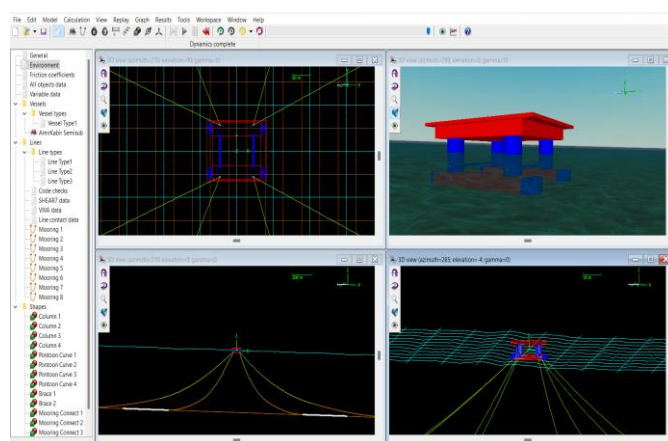
شکل ۱۴ - مدل سکوی نیمه شناور امیر کبیر
