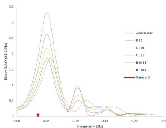
شکل ۱۸ - نمودار مقایسه و بررسی طیف دامنه پاسخ حرکت هیو
