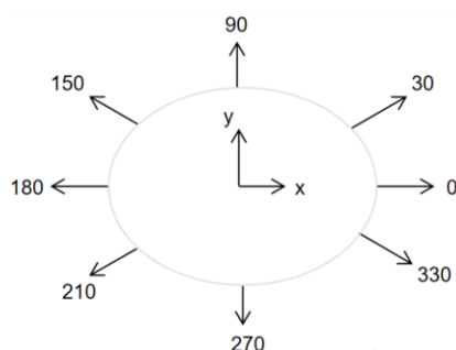
شکل ۱۱- زوایای نیرو و مهار در مدل‌ها
