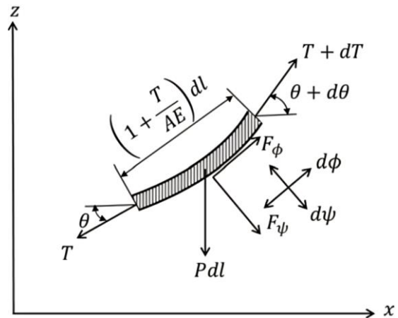
شکل ۵- نیرو و جابجایی روی یک عنصر از خط مهار [۱].
