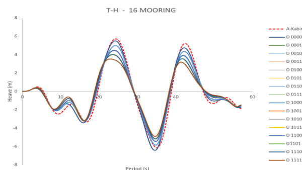
شکل ۱۵ - حرکت هیو سکو در مدل‌های ۱۶ مهاري گام اول
